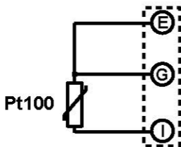
3 wires Pt100
