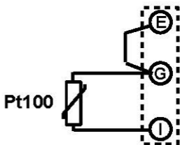
2 wires Pt100
